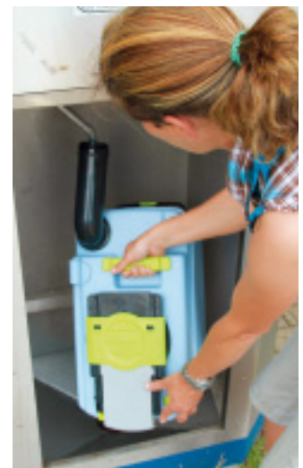
Pfiffig gelöst: Weit entfernt vom Frischwasseranschluss öffnet sich der Rollladen und gibt den Schacht frei. Das Spülen würde etwas einfacher gelingen, wenn das Spülrohr weiter vorn platziert wäre.
