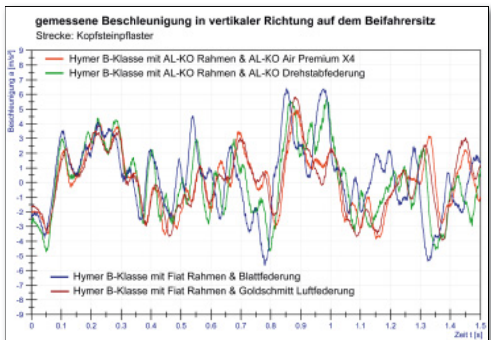
In diesem Schaubild sind die Messwerte exakt der gleichen Fahrstrecke übereinandergelegt. Je geringer die Ausschläge der Kurven, desto komfortabler ist das Fahrwerk. Die beiden luftgefederten Fahrwerke haben an der Vorderachse die Nase vorn.
