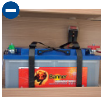
Die Pole der ungeschützten Batterie stehen frei: Kurzschlussgefahr.
