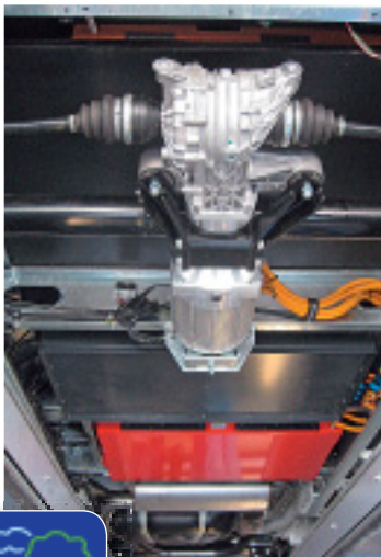
Blick von unten auf die B-Klasse. Rot die Batterie, vorn Motor, Differenzial und Antriebswellen.
