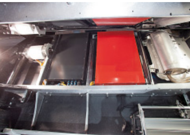
Ein großer Spiegel ermöglicht den Blick unter das Mobil und offenbart das Electric Power Chassis von Al-Ko.
