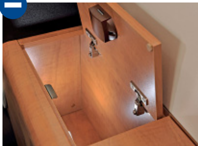
Scharfkantige Metallschließbleche in den Cockpitablagen montiert.
