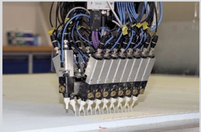
Exakter und sparsamer als manuelles Aufbringen mit dem Rechen: Vollautomatisch verteilt die Maschine bei Carthago den Kleber auf den Bauteilen. Aus Innenschicht, Isolierung und Außenschicht entstehen Wände, Böden und Dächer.
