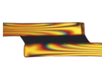
Bei der elastischen, dickschichtigen Klebeverbindung verteilen sich die Kräfte optimal gleichmäßig.
