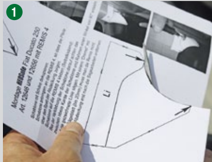
1 Selbstklebende Schneideschablone ausschneiden und auf die Ecke der Remis 4 aufkleben
