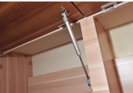
Sauber gemacht: Die Klappen der Oberschränke bekommen solide Teleskopaufsteller mit auf den Weg, die Tischverbreiterung wird sicher im Kleiderschrank untergebracht.
