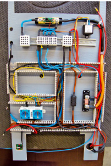
Montagefreundlich: Das Elektronik-Paket für die Platin-Edition können die Monteure im Werk übersichtlich und bequem auf der Werkbank vorinstallieren. Ein Schmuckstück: das Elektro-Paket fertig im Fahrzeug installiert.
