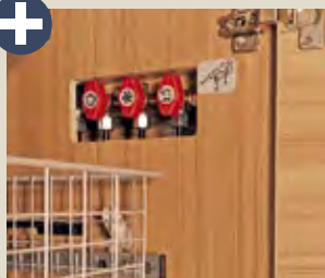
In Stehhöhe installiert, sind die Gas- absperrhähne leicht zu bedienen.
