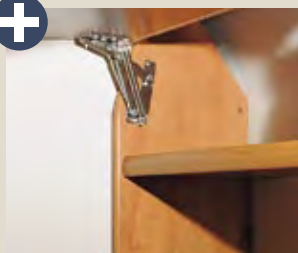
Hochwertige Metallscharniere schließen tadellos.
