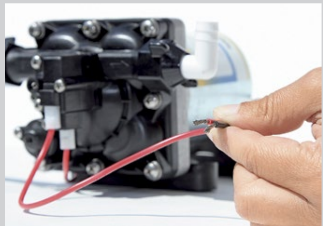
Kabelquerschnitt: Für den Anschluss der Pumpe an die Bordbatterie empfehlen Experten einen Kabelquerschnitt von vier Quadratmillimetern. Vorausgesetzt, die Leitungen sind nicht länger als sechs Meter. Bei noch längeren Kabeln sollte der Kabelquerschnitt auf sechs Quadratmillimeter wachsen.
