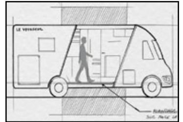
Keine Stufe im Aufbau dank des durchgehenden, vollwertigen und 26 cm hohen Doppelbodens
