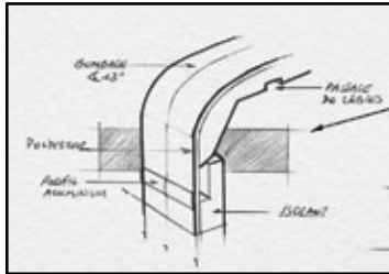
Gebogenes GFK-Dach bis über die Seitenwände für optimalen Wasserablauf
