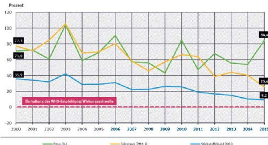
Abstand der durchschnittlichen Schadstoffkonzentrationen zu WHO-Empfehlungen* bzw. festgestellten Wirkungsschwellen** im städtischen Hintergrund deutscher Ballungsräume
