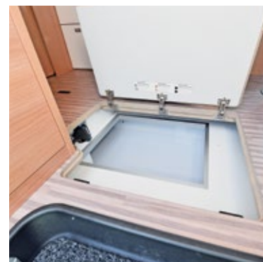
Stabile Klappen öffnen den Doppelboden für sperriges Gepäck. Hier finden sich auch die vorbildlich beschrifteten Ablasshähne.
