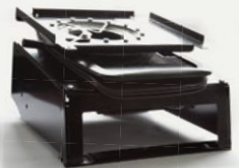
Abb.: Luftfederung und Drehkonsole auf niederem Aguti-Sitzkasten
