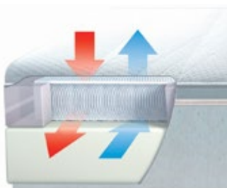
Die Matratze Vital von Hersteller Gisamed im Querschnitt: oben das luftige Dryweave samt atmungsaktiver Auflage, unten die Kaltschaumbasis.
