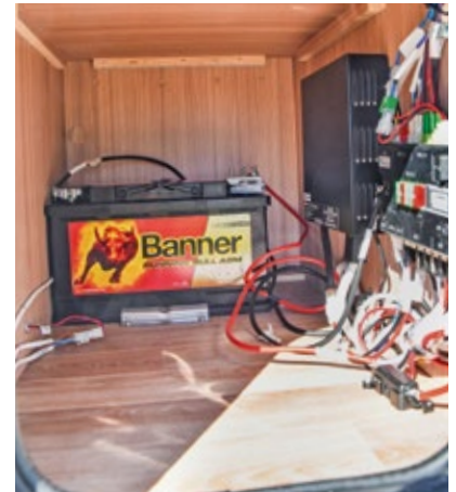
Licht und Schatten: Der WC-Schacht ist sehr gut abgedichtet. Die Kabel im Service-Fach sollte Ahorn sorgfältiger verlegen.
